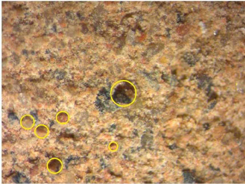
Porosidad de mortero 12.5M KOH
