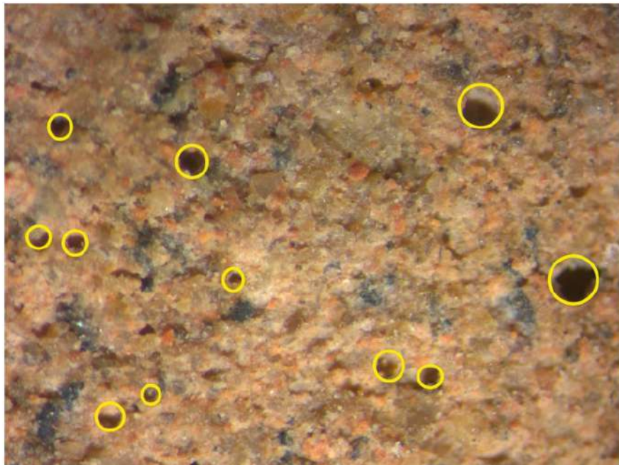
Porosidad de mortero 7.5M KOH
