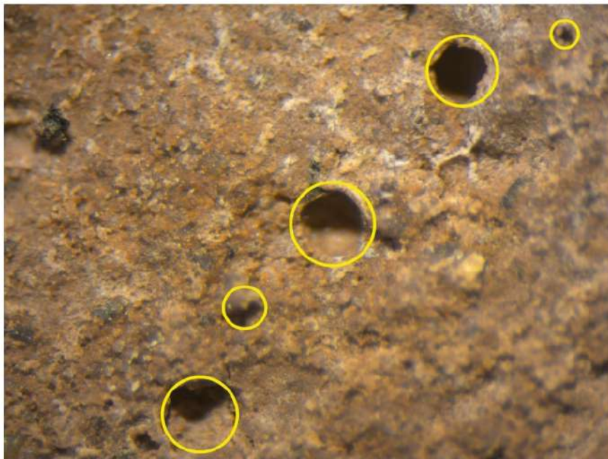
Porosidad de mortero grupo control
