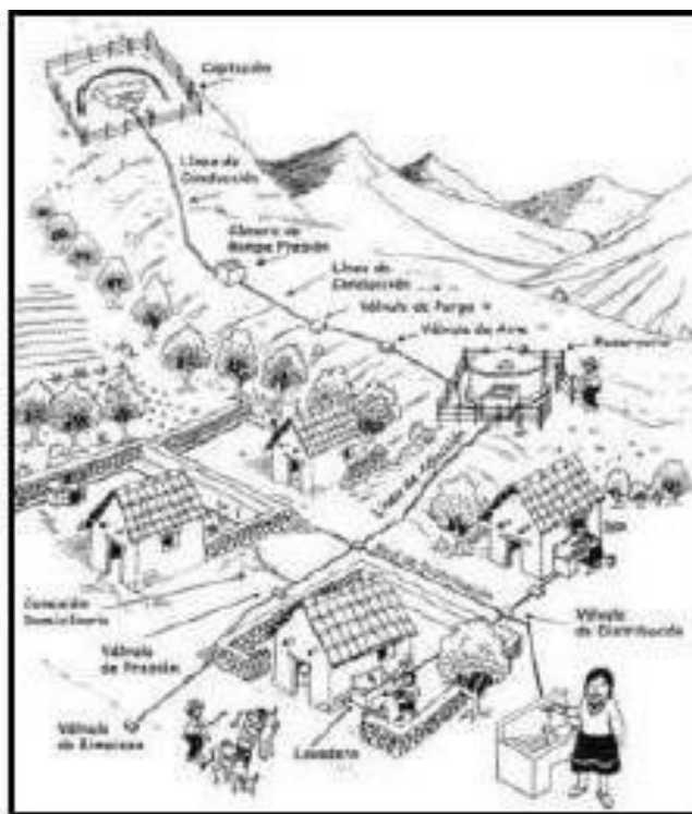
Figura 01: Componentes de un abastecimiento de agua potable.
