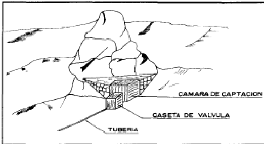
Figura 05: Captación de agua subterránea (manantial)
