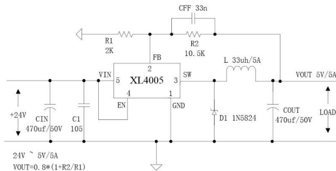
Figura 10. Diagrama del regulador XL 4005
