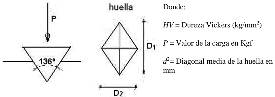
Gráfico 2. Diagrama de ensayo de dureza Vickers (Fullmecanica. 42 2014)
